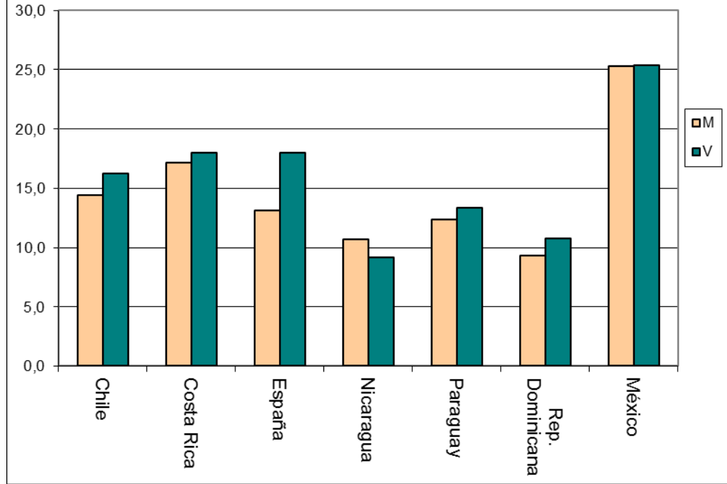
Antigüedad media por país y sexo
